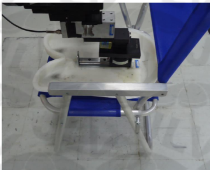
FOTO 2: AMOSTRA DURANTE O ENSAIO
